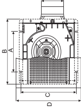
BPT10-13H20, BPT10-23H25, BPT10-23H30 BPT10-23H35, BPT15-33H45, BPT15-33H55
