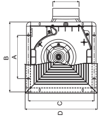
BPT10-13H20-A, BPT10-23H25-A, BPT10-23H30-A BPT10-23H35-A, BPT15-33H45-A, BPT15-33H55-A
