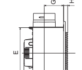
BPT10-13H20-T, BPT10-23H25-T, BPT10-23H30-T BPT10-23H35-T, BPT15-33H45-T, BPT15-33H55-T
