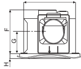
BPT10-13H20, BPT10-23H25, BPT10-23H30 BPT10-23H35, BPT15-33H45, BPT15-33H55
